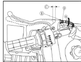
1. Contraporca 2. Parafuso de ajuste c. Espaçamento do manete de freio traseiro
