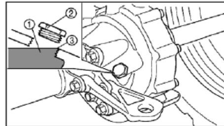
1. Óleo da marcha final 2. Parafuso do reservatório de óleo da marcha final 3. Nível de óleo adequado
