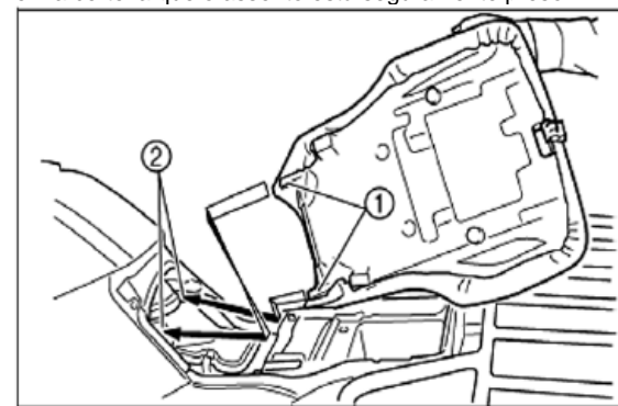
1. Projeção (×2) 2. Ganchos do assento (×2)
